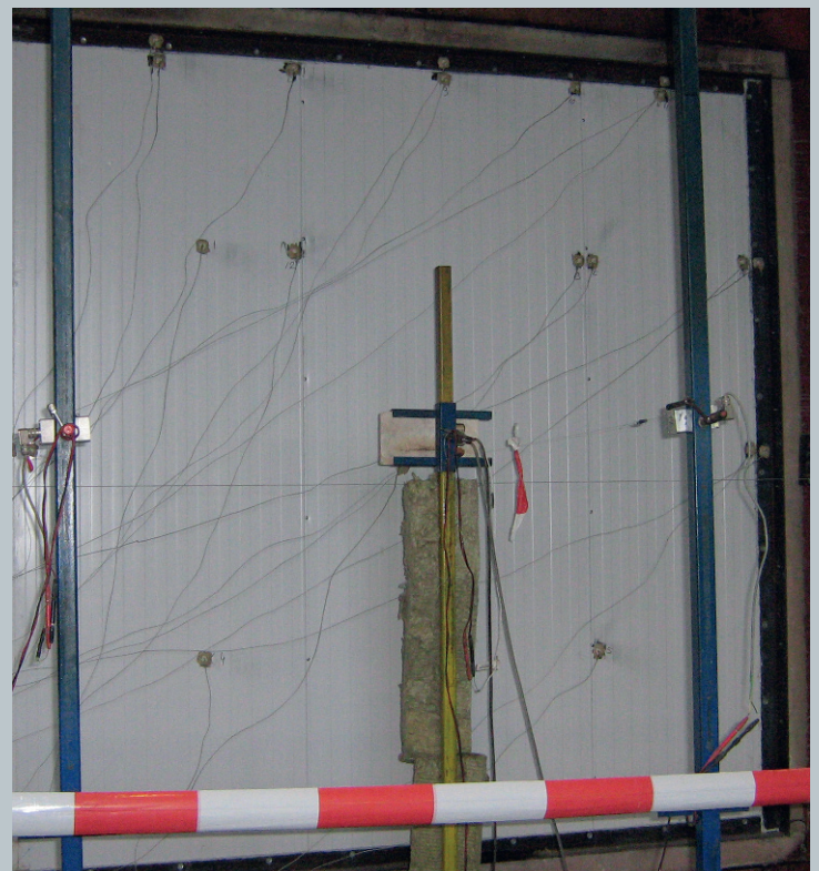
Kingspan-brandtest door Efectis.
